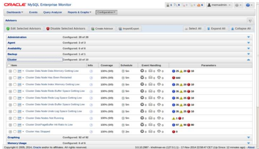
Figure 3. Les conseillers experts MySQL Cluster recommandent les meilleures pratiques et réduisent les risques de temps d'arrêt
