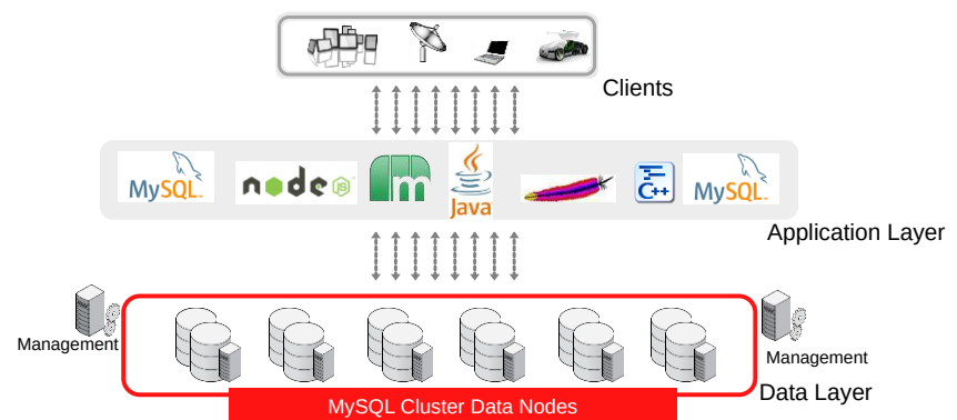
Figure 1. L'architecture MySQL Cluster est conçue pour une évolutivité élevée et une disponibilité de 99,999 % avec des API SQL et NoSQL
